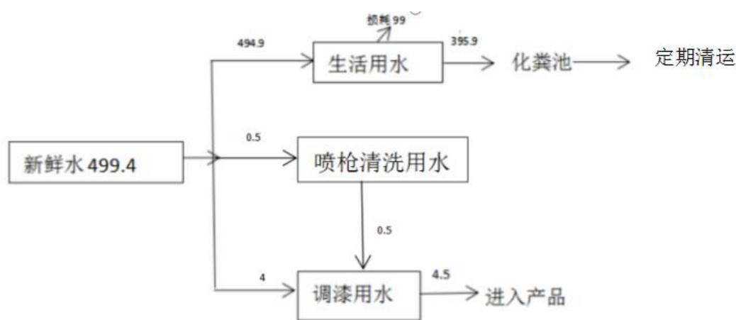
图3-1 本项目水平衡图 (t/a)
